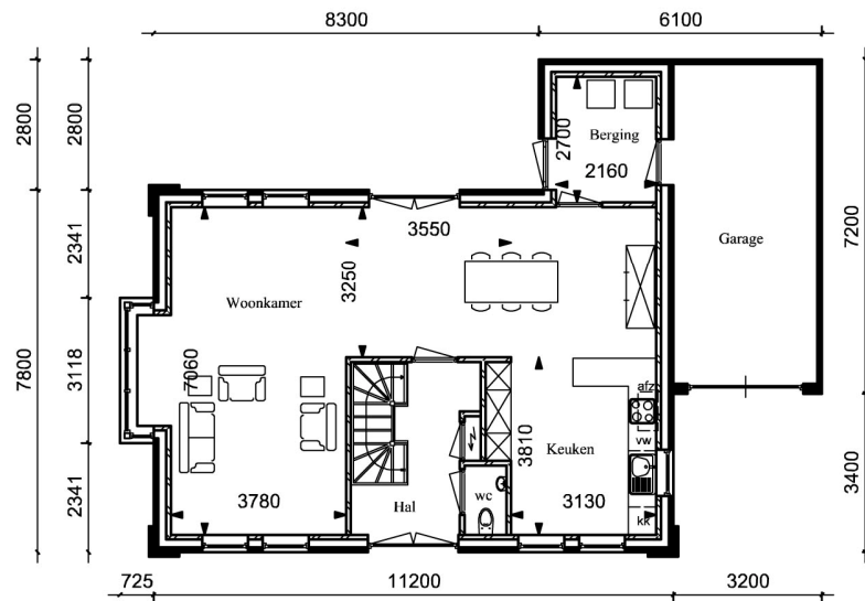
Begane grond. _____
